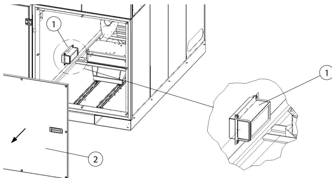
Rys. 40: Dostęp do filtra zabezpieczającego
