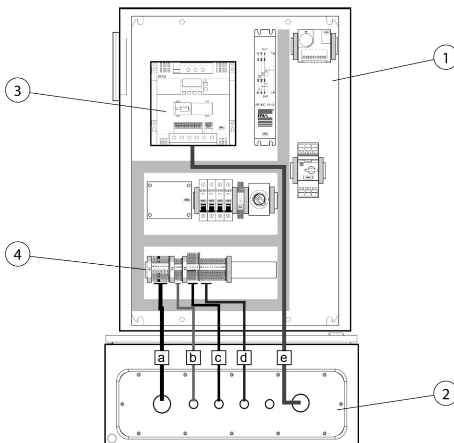
Rys. 16: Szafa rozdzielcza, układ regulacji mocy ssącej
